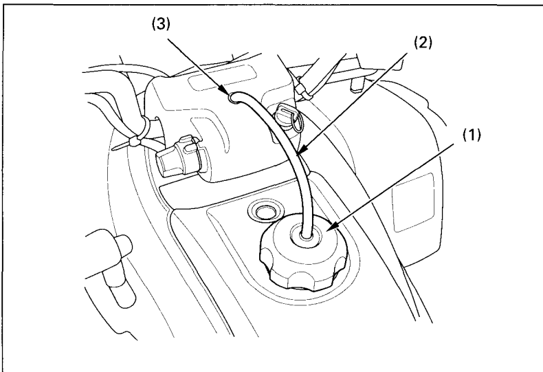
Fig. 2-28 (1) Fuel fill cap
