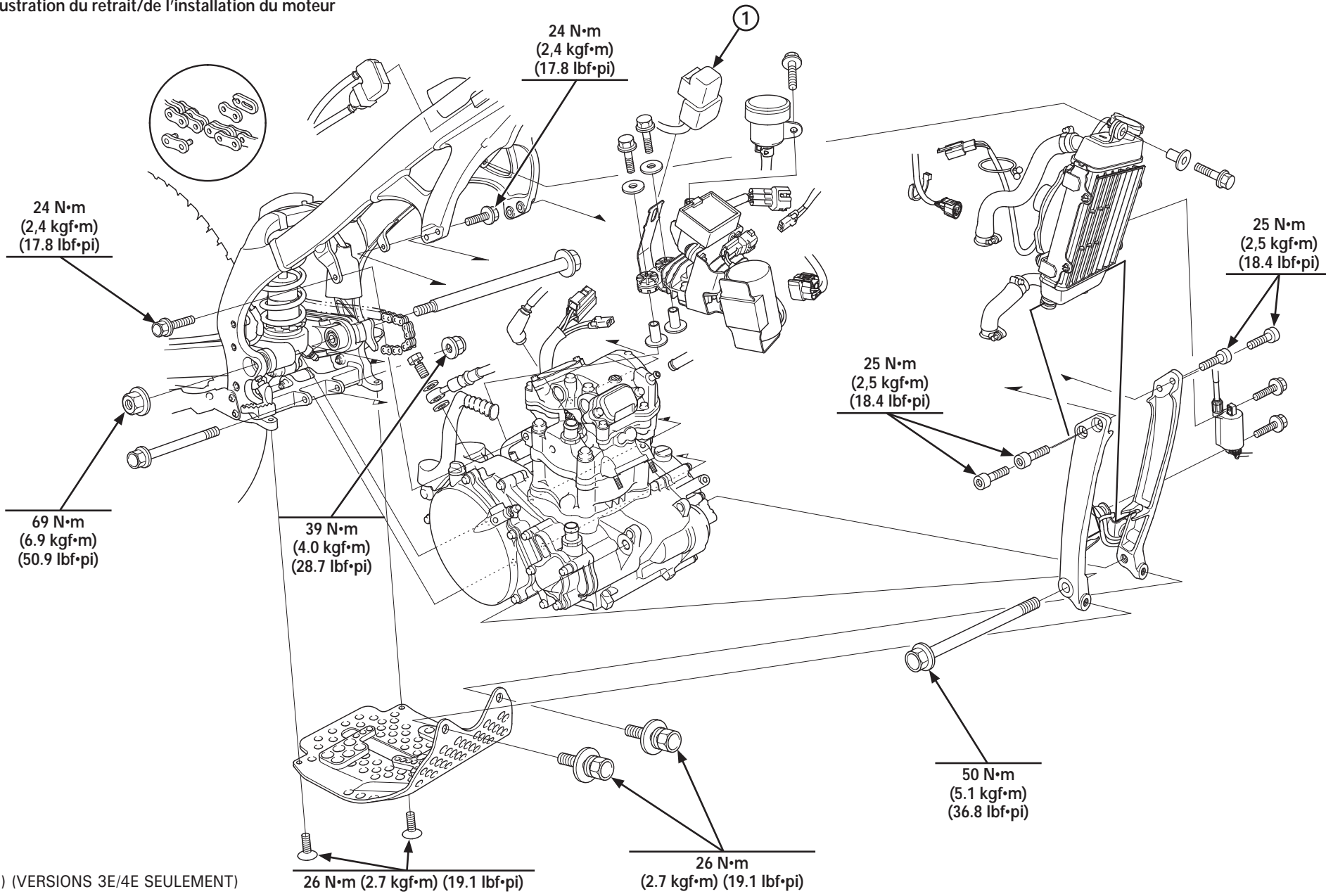
Illustration du retrait/de l'installation du moteur
