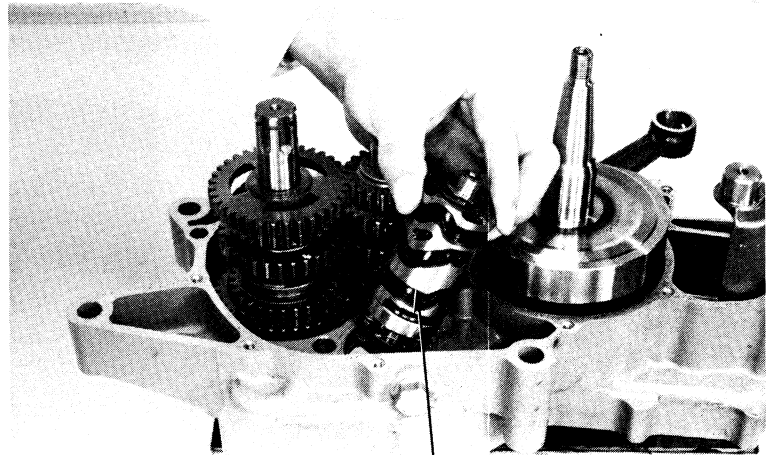
SHIFT DRUM
