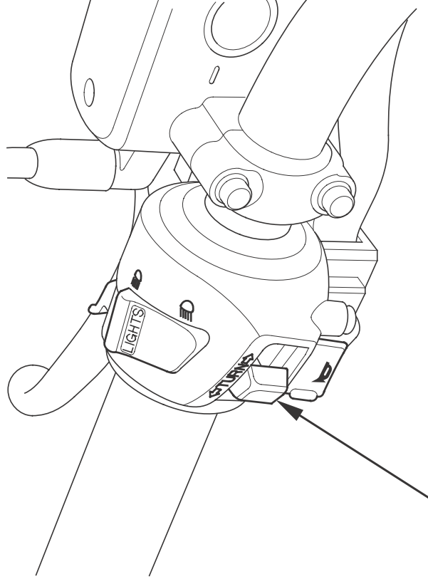
方向指示器スイッチ
