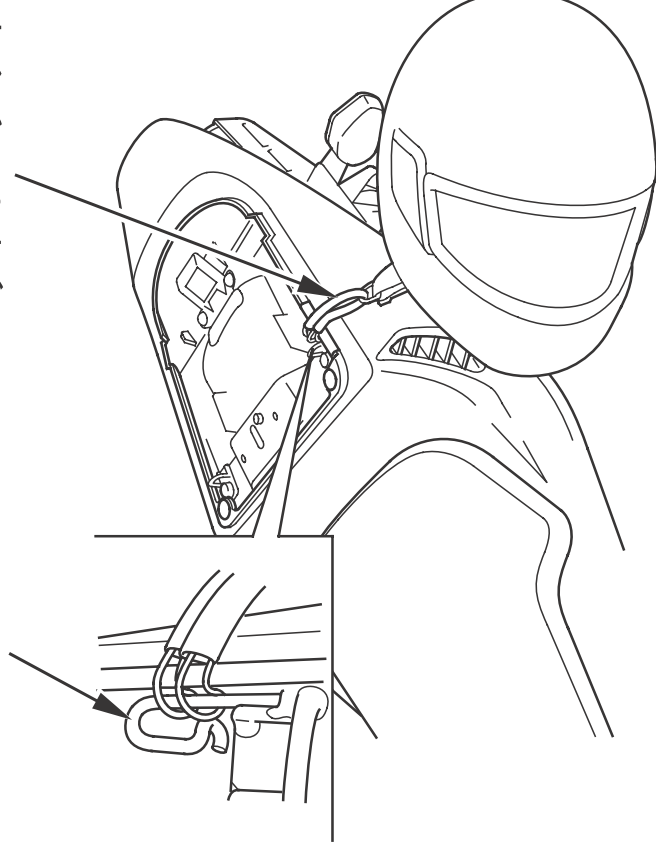
ヘルメットホルダ ヘルメットホルダワイヤ
