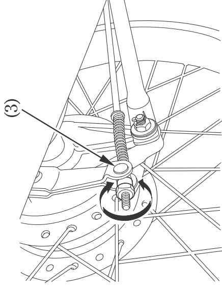
(3) Pasador del brazo del freno
