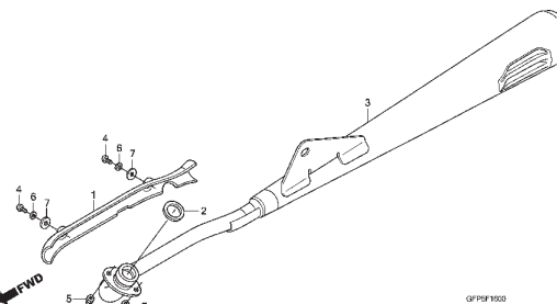
C-16 Escapamento / Exhaust Muffler / Silenciador
