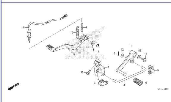
C-29 Pedal
